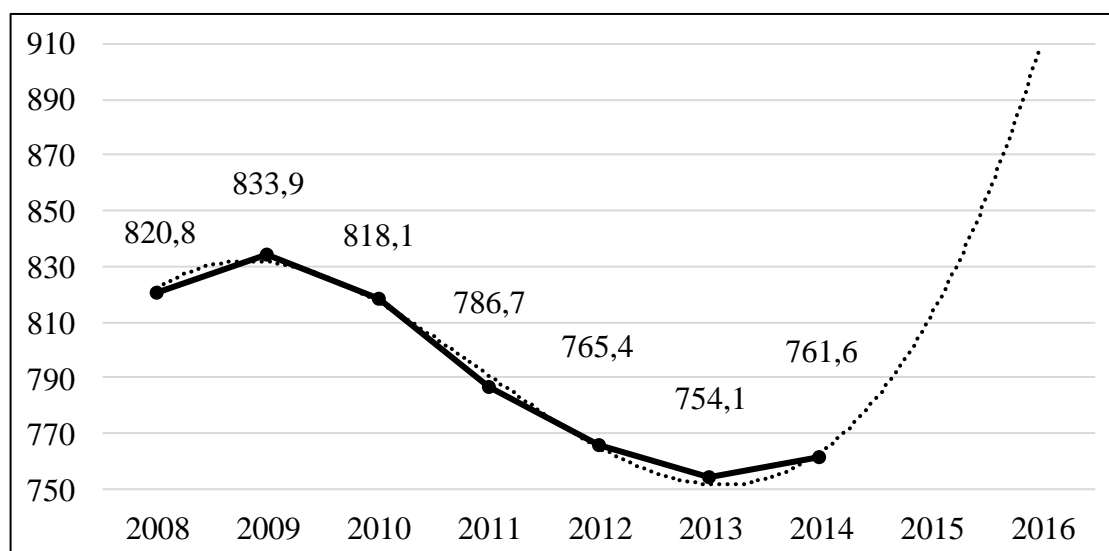
Рис. 1. Прогнозирование численности населения РФ на конец 2016 года на основе тренда, тыс. человек.
